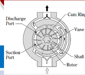
تیغه‌ای دورانی
