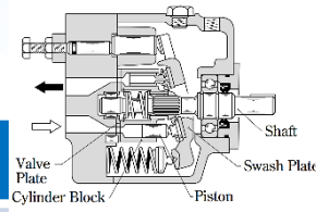
پیستونی
